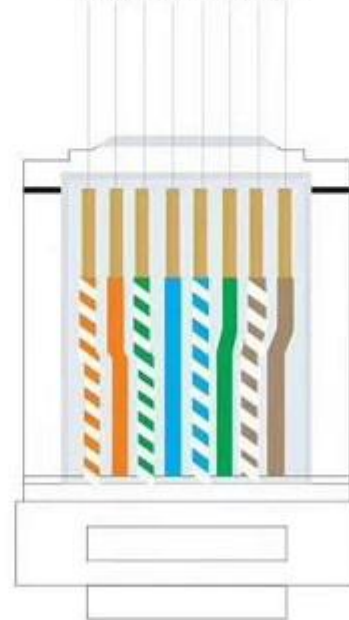
T568B标准
