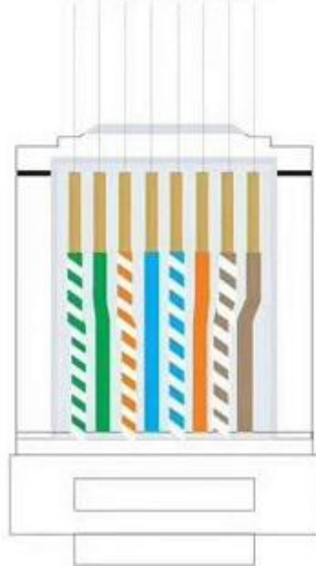
T568A标准
